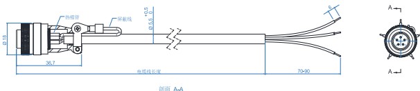
剖面 A-A
